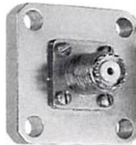
Mini-UHF (F) 4240-346
